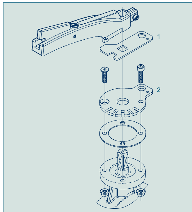
1 - Проушина 2 - Растровая пластина с проушиной под пломбу
